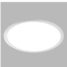
EASY-R L 18W 3000K/4000K 1620 lm/1800 lm
